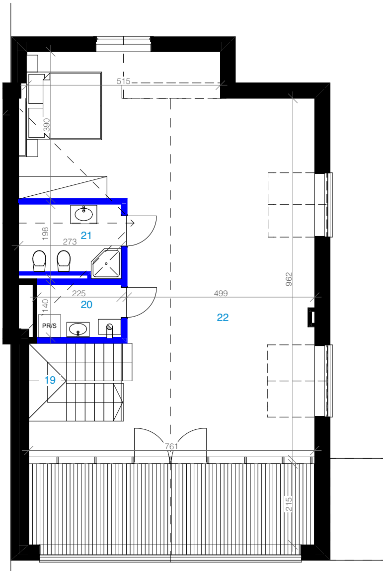
Rzut poddasza 1:100
